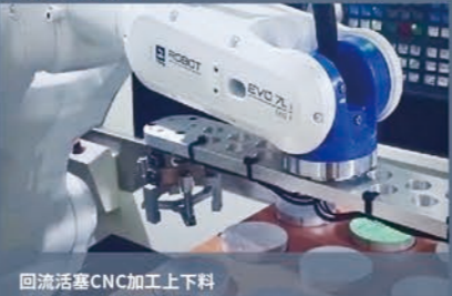
回流活塞CNC加工上下料 型号:EVO7L
