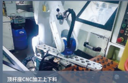
顶杆座CNC加工上下料 型号:EVO7L
